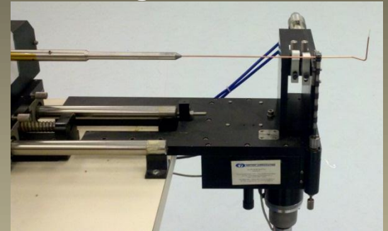
Semi-rigid Auto-bender
